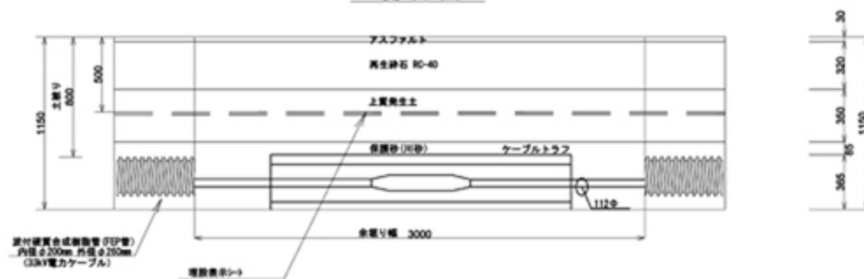
側面図
